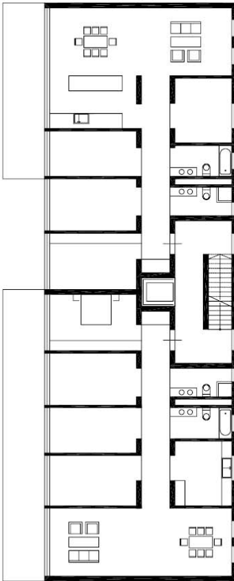
Grundriss Obergeschoss 1:200
